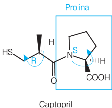
Figura 18: Pedacos do captopril.
