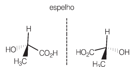
os enantiômeros do ácido láctico
