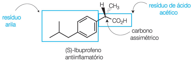
Figura 17: Pedacos do ibuprofeno.
