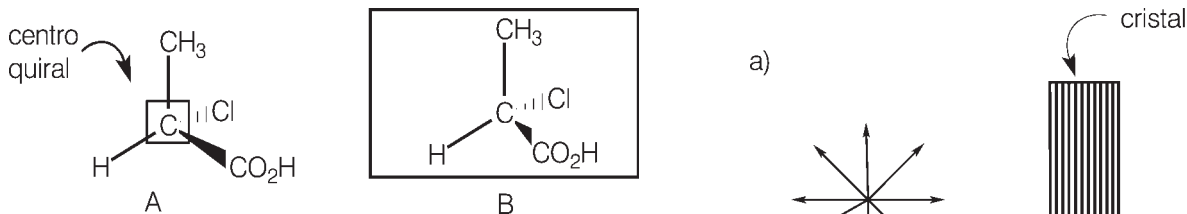
Figura 8: Representações de um centro assimétrico.
