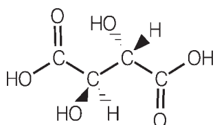
Figura 1: Estrutura do ácido (+)-tartárico.
