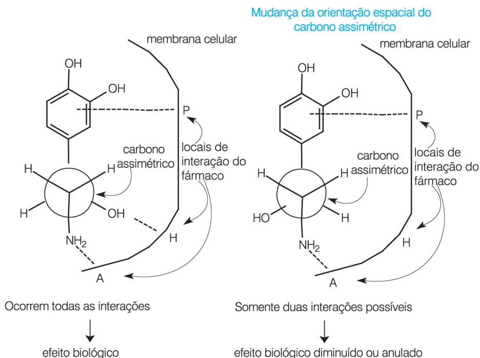
Figura 15: Aplicação do modelo à noradrenalina.
